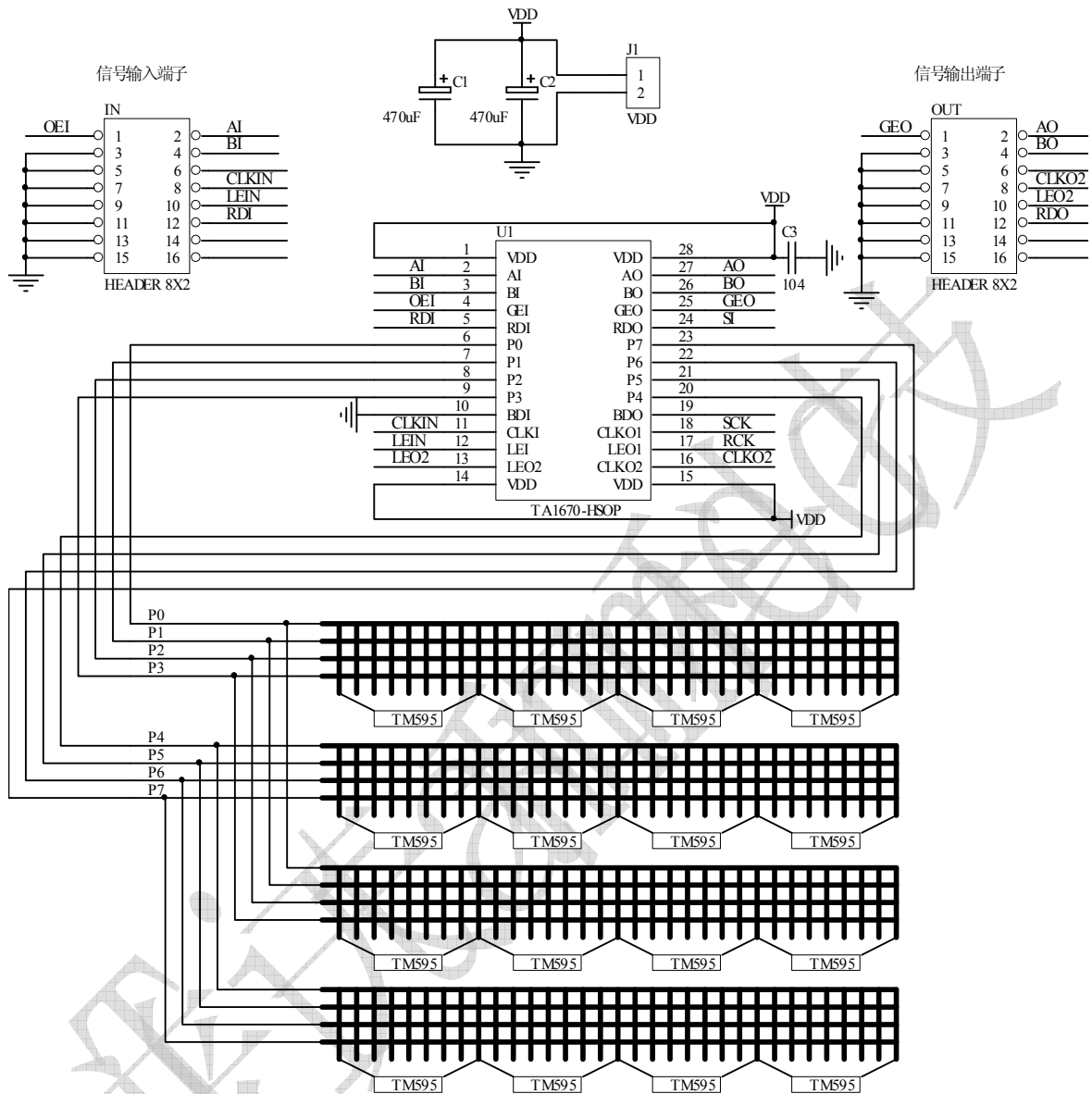
32×16 LED点阵 图六 P10 方案接线原理图
